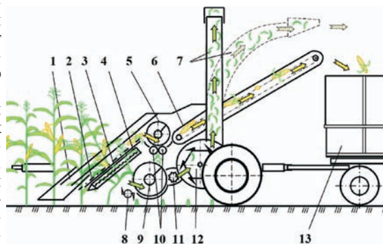
Такмиллаштирилган маккажўхори йиғиш машинаси схемаси
