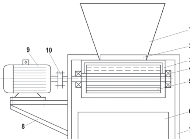
1-юклар бункери; 2-уруғ меъерини ростлайдиган мослама; 3-ҳаво оқимининг тезлигини ростлайдиган мослама; 4-подшипниклар; 5-вентилятор; 6-қабул қилиш бункери; 7- рама; 8- асос; 9- электродвигатель; 10-муфта.
